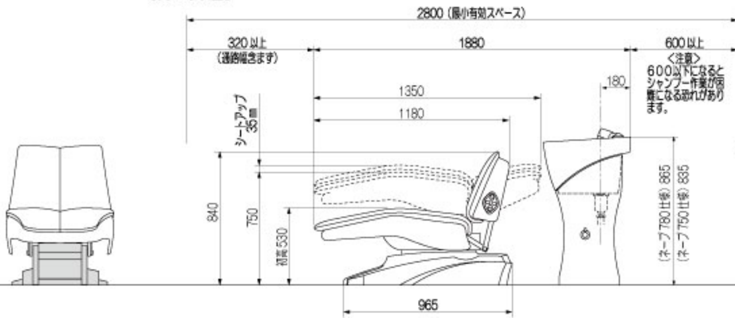
【側面寸法図】
